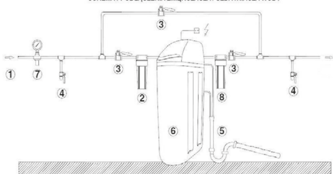
SCHEMAT PODŁĄCZENIA ZMIĘKCCZACZA / UZDATNIACZA WODY
